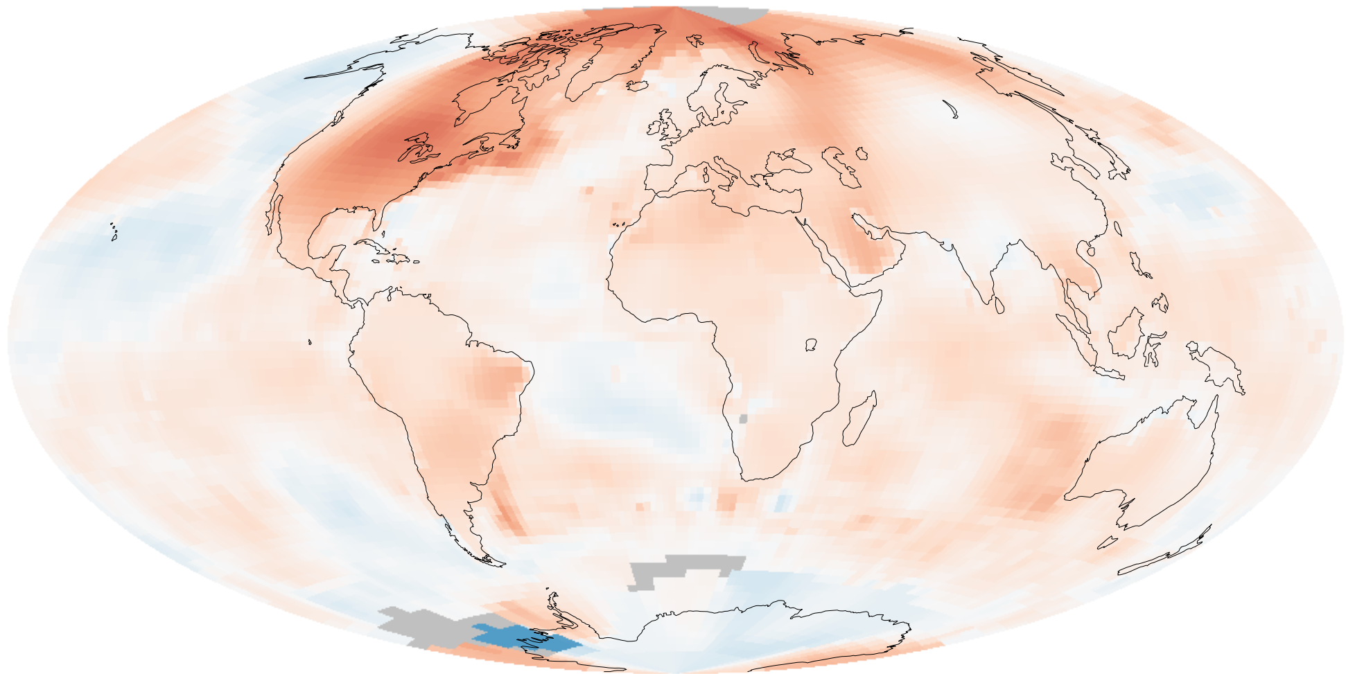
2012 Global Temperature Anomaly(°C)
